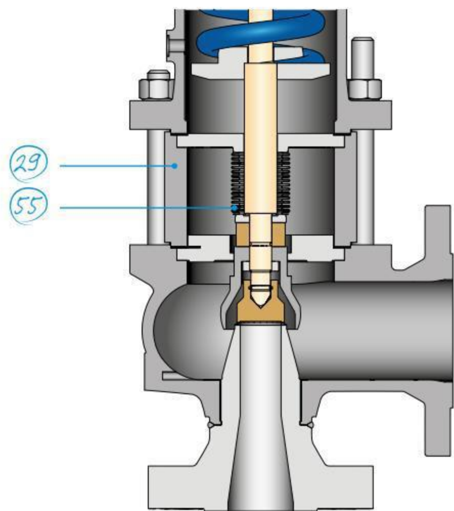
Bellows design Si 6403
