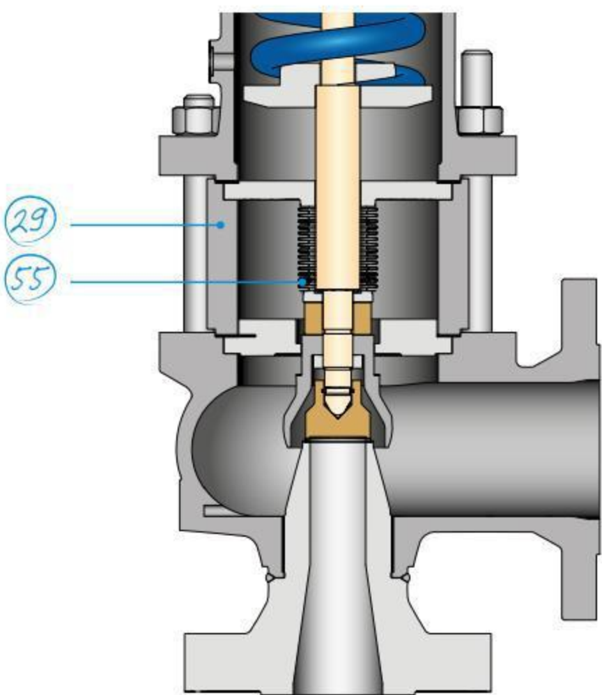
Bellows design Si 6404
